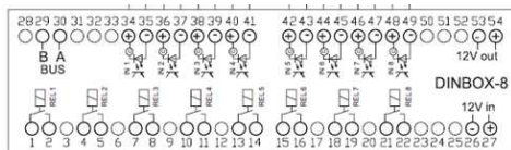
Styringskort ems-1080
